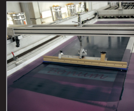
De inkt wordt nu door de zeefgaatjes gedrukt op het glasopper-vlak. Dit proces herhaalt zich met elke kleur.
